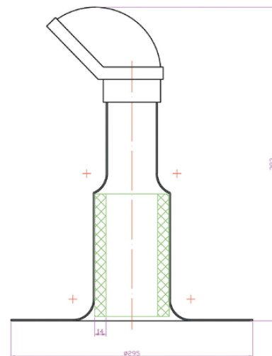
Fig. 1. Solin d'étanchéité isolé pour fils électrique
